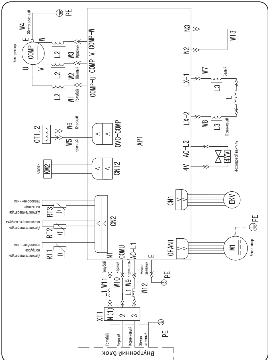
Схема электрическая наружного блока.
